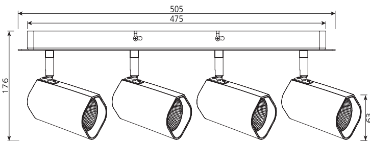
B-Quad
